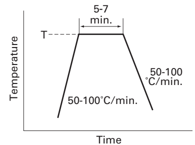
Fig. 2 L/A profile
