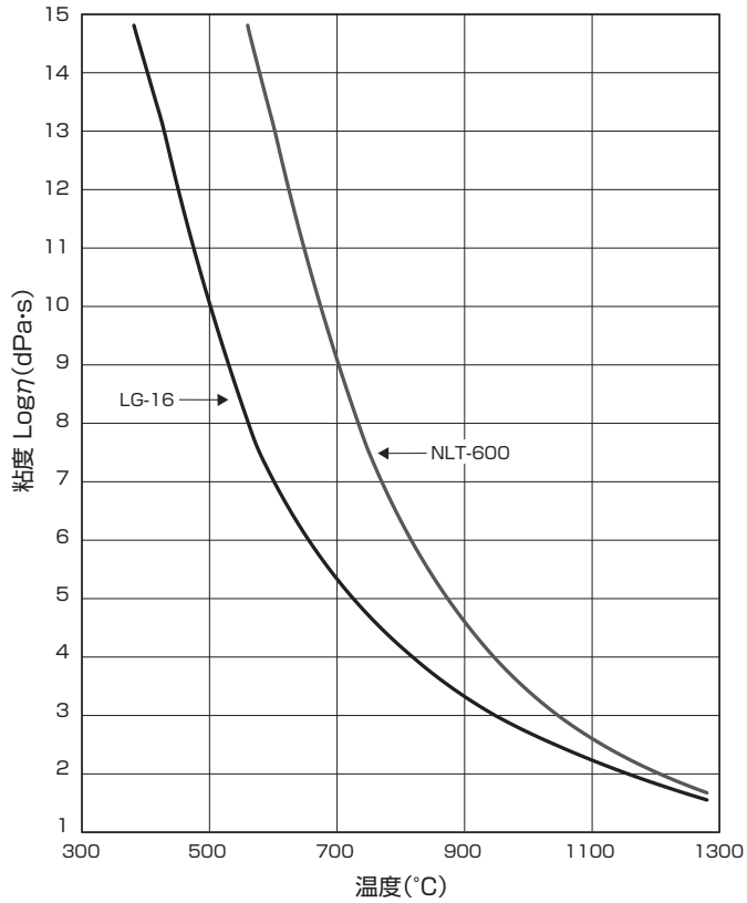
粘度曲線
