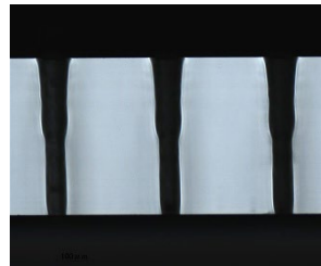
CO 2 レーザーによる ガラス基板写真（上）とその断面写真（下） （基板厚み 0.5mm、穴径Φ90μm）
