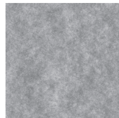
G-Leaf® オーバーフロー法(未研磨品) Ra=0.2nm
