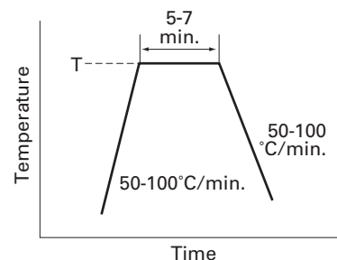
Fig. 2 L/A profile
