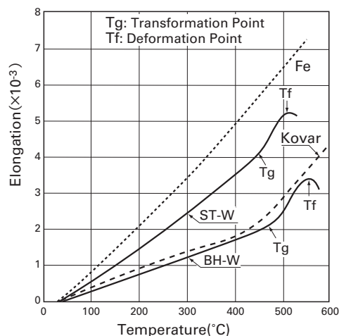
Fig. 4 Thermal expansion
